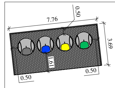
Aikštelės detalizacija
